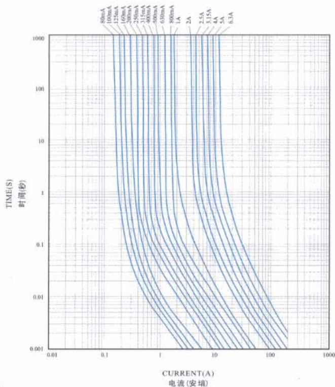
I-T CHARACTERISTICS CURVE 电流-时间曲线图
