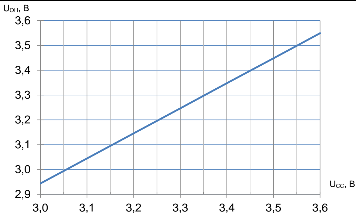
Рисунок 41 – Зависимость выходного напряжения высокого уровня от напряжения питания при I_{OH} = \text{минус } 2 \text{ мА} , T = 25 \text{ }^\circ\text{C}
