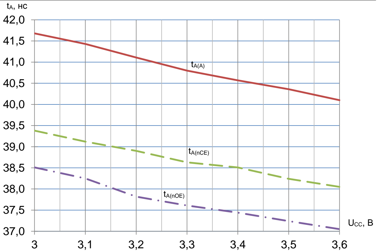
Рисунок 45 – Зависимость времени выборки адреса t_{A(A)} , времени выборки по сигналу nCE t_{A(nCE)} , времени выборки по сигналу nOE t_{A(nOE)} от напряжения питания при T = 125\text{ °C}
