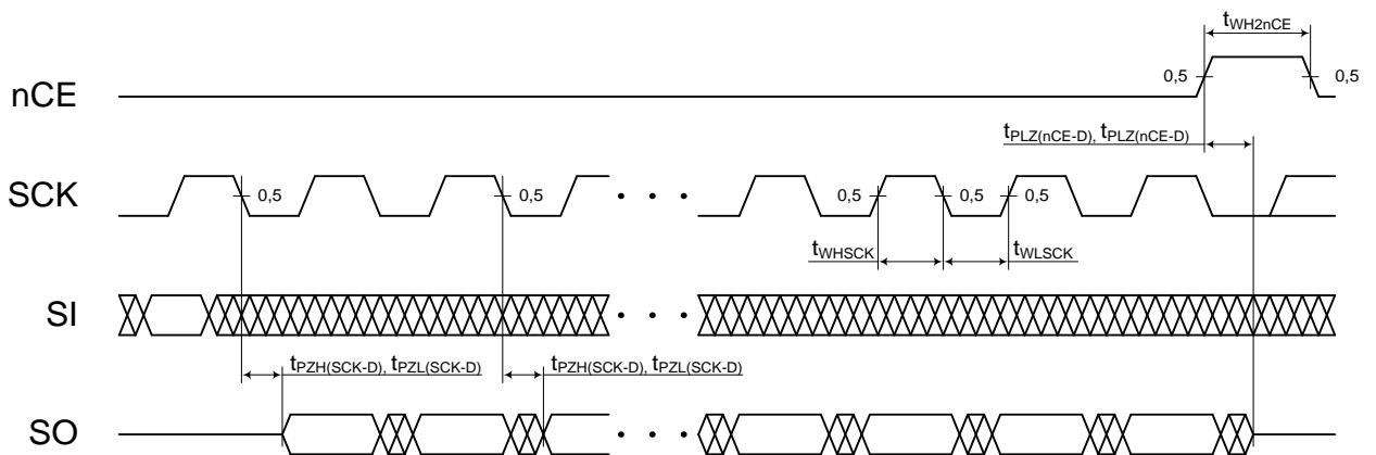
Рисунок 36 – Временная диаграмма чтения последовательного канала SPI
