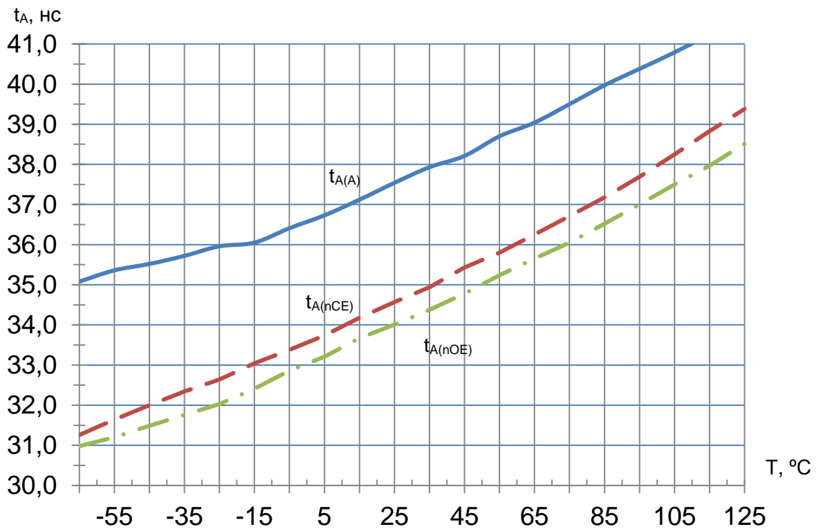
Рисунок 46 – Зависимость времени выборки адреса t_{A(A)} , времени выборки по сигналу nCE t_{A(nCE)} , времени выборки по сигналу nOE t_{A(nOE)} от температуры при U_{CC} = 3,0\text{ В}
