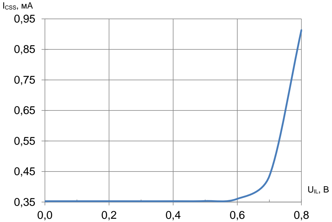
Рисунок 39 – Зависимость тока потребления в режиме хранения от входного напряжения низкого уровня при U_{CC} = 3,6 В, U_{IH} = 3,6 В, f = 0 МГц, T = 25 °С
