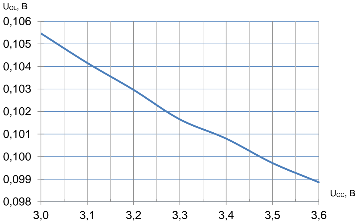
Рисунок 40 – Зависимость выходного напряжения низкого от напряжения питания при I_{OL} = 4 мА, T = 25 °С
