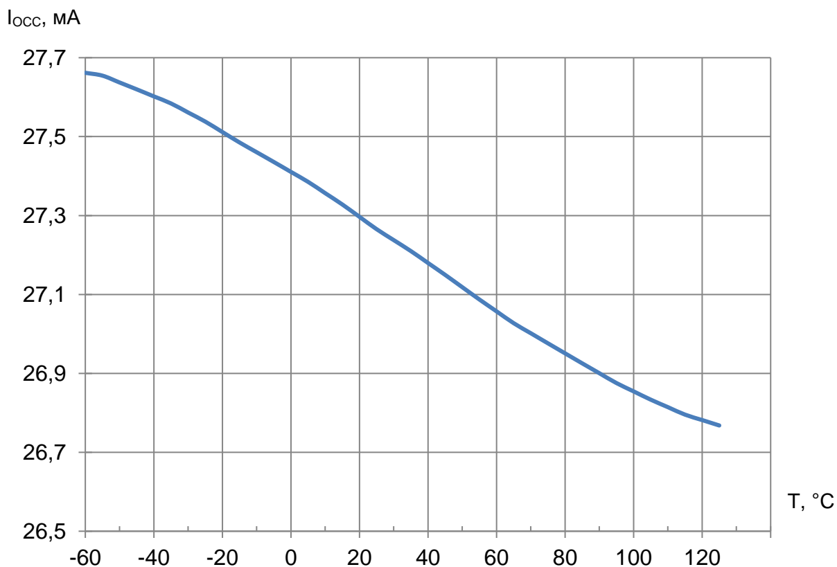
Рисунок 42 – Зависимость динамического тока потребления от температуры при U_{CC} = 3,6 \text{ В} , t_{CYR} = 70 \text{ нс}
