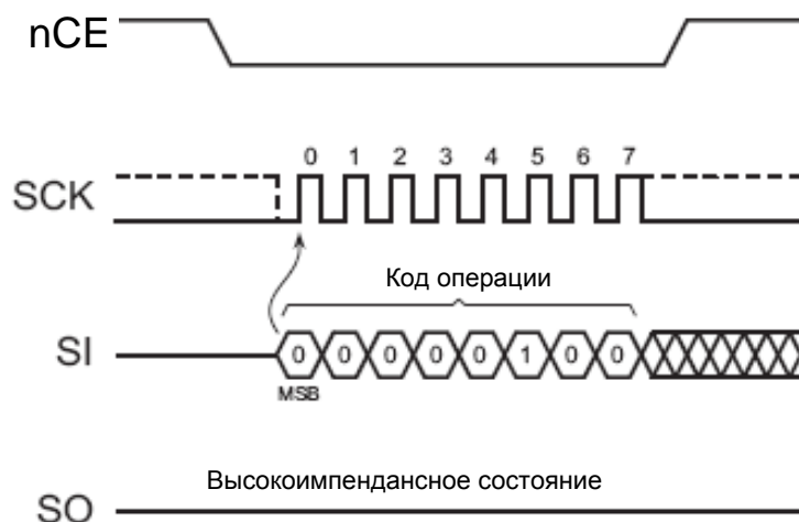
Рисунок 20 – Операция запрета записи
