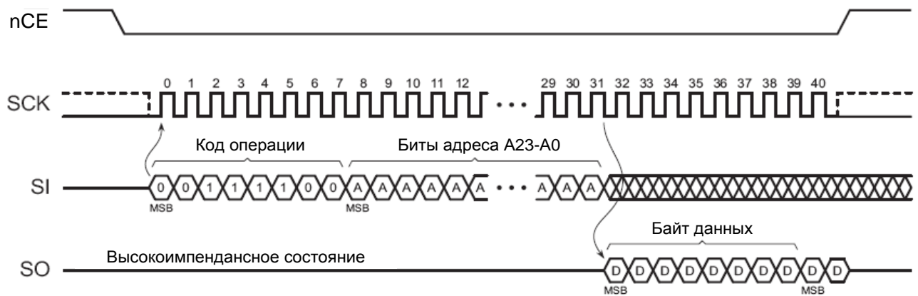
Рисунок 23 – Операция чтения регистра защиты сектора
