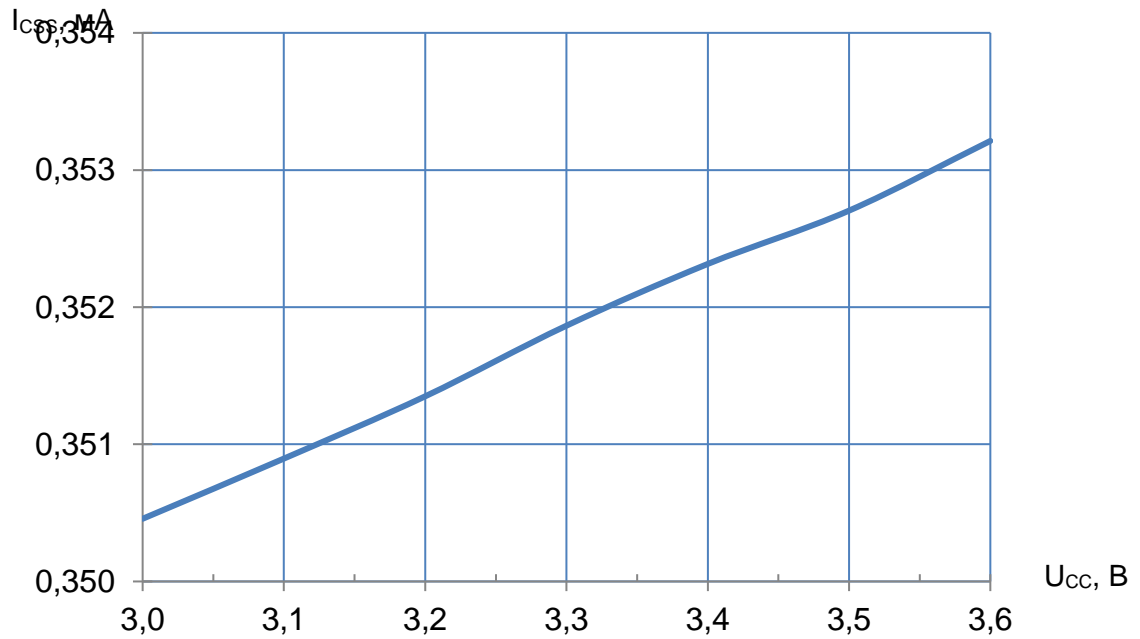
Рисунок 37 – Зависимость тока потребления в режиме хранения от напряжения питания при T = 25\text{ }^{\circ}\text{C}
