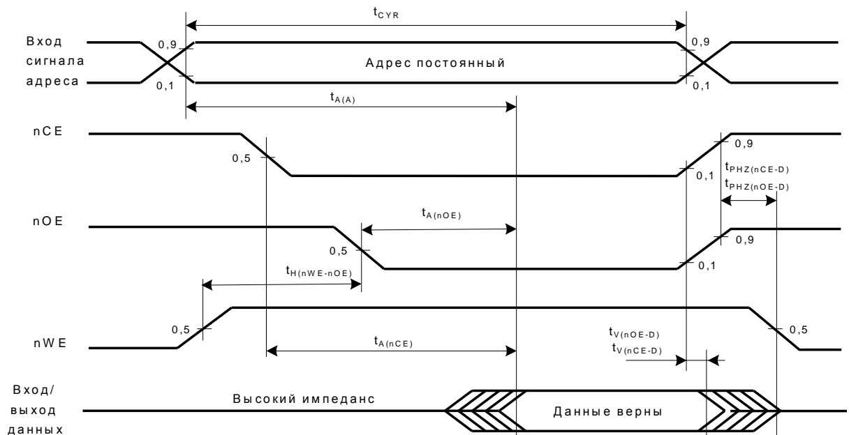
Рисунок 29 – Временная диаграмма цикла чтения 2. Управление по nOE, nCE. U_{nWE} = U_{IH} . Сигналы на выводах TDI, TCK, STROBE в состоянии логической «0», MRST логической «1»
