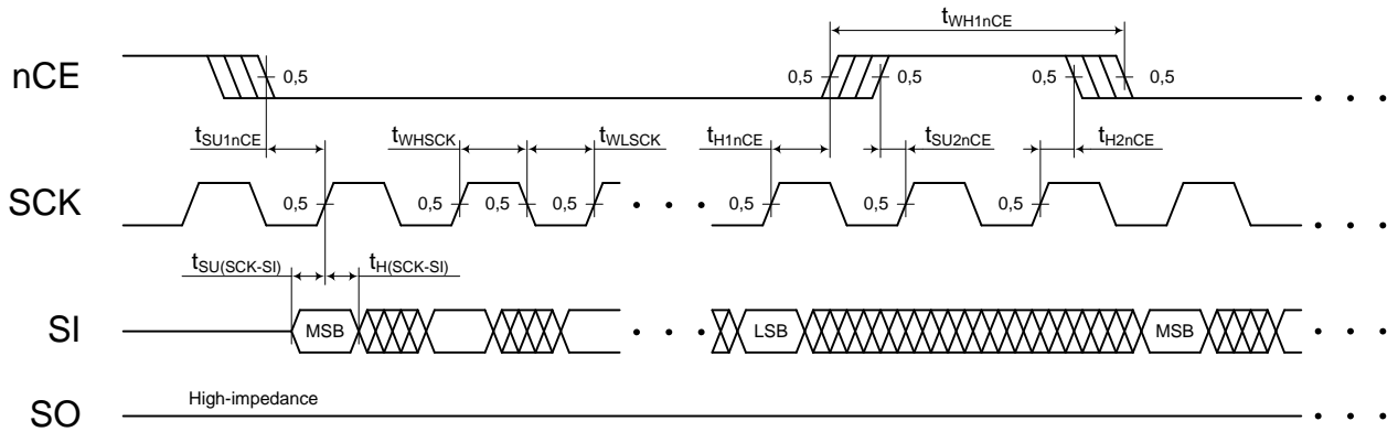
Рисунок 35 – Временная диаграмма записи последовательного канала SPI
