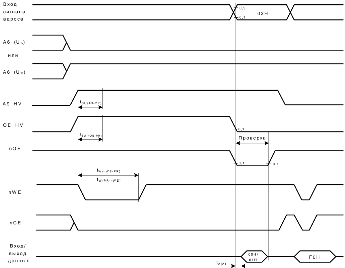
Рисунок 32 – Временная диаграмма цикла защиты/снятия защиты
