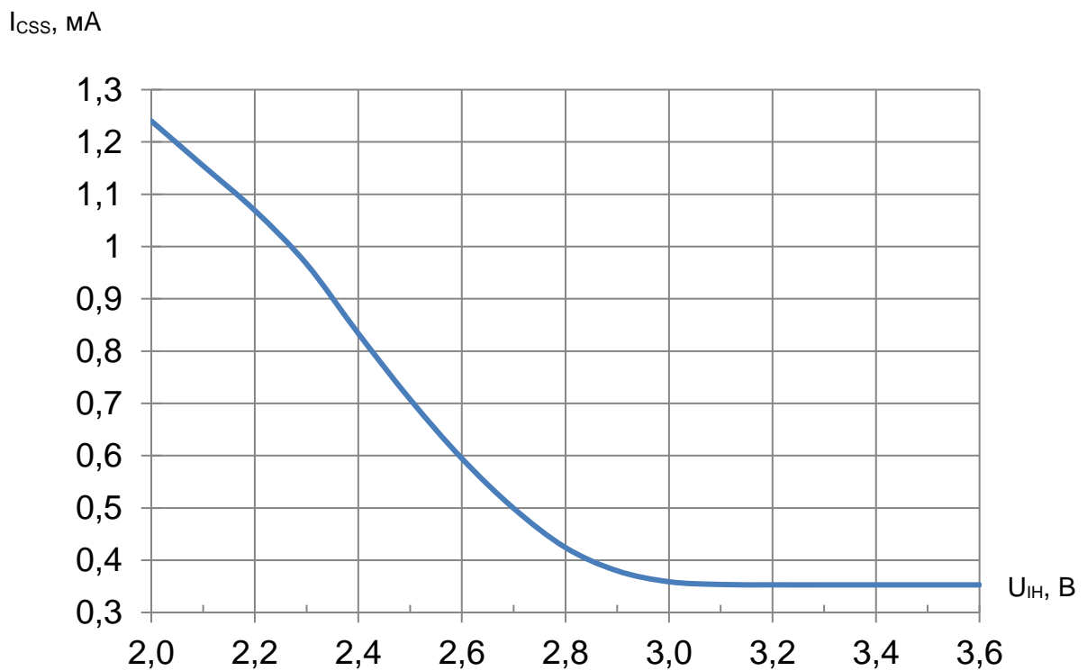
Рисунок 38 – Зависимость тока потребления в режиме хранения от входного напряжения высокого уровня при U_{cc} = 3,6\text{ В} , U_{IL} = 0\text{ В} , f = 0\text{ МГц} , T = 25\text{ }^{\circ}\text{C}
