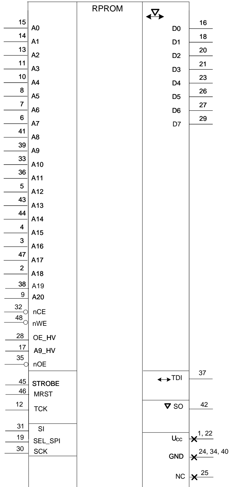
Рисунок 2 – Условно-графическое обозначение
