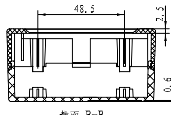
截面 B-B
