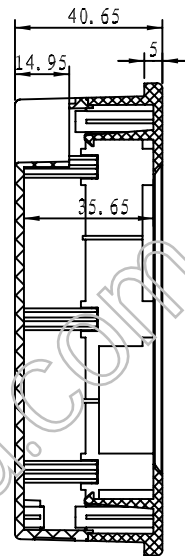
截面 A-A
