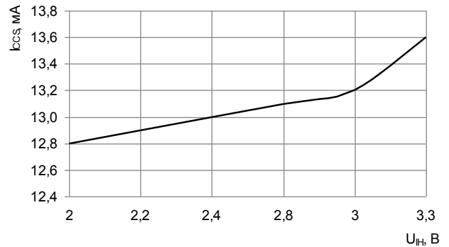
Рисунок 20 – Зависимость тока потребления в режиме хранения, от входного напряжения высокого уровня
