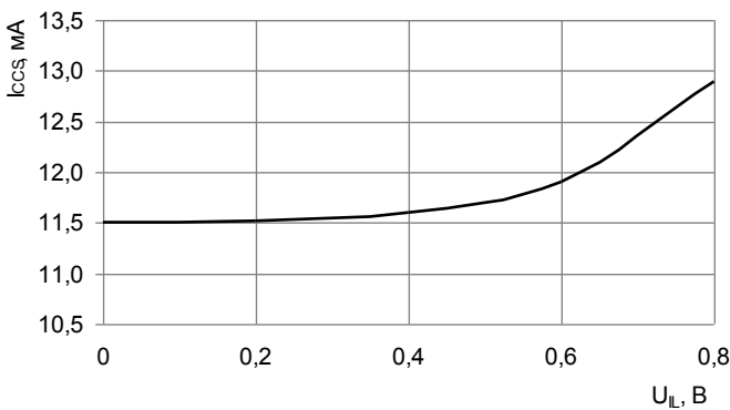
Рисунок 21 – Зависимость тока потребления в режиме хранения, от входного напряжения низкого уровня,
