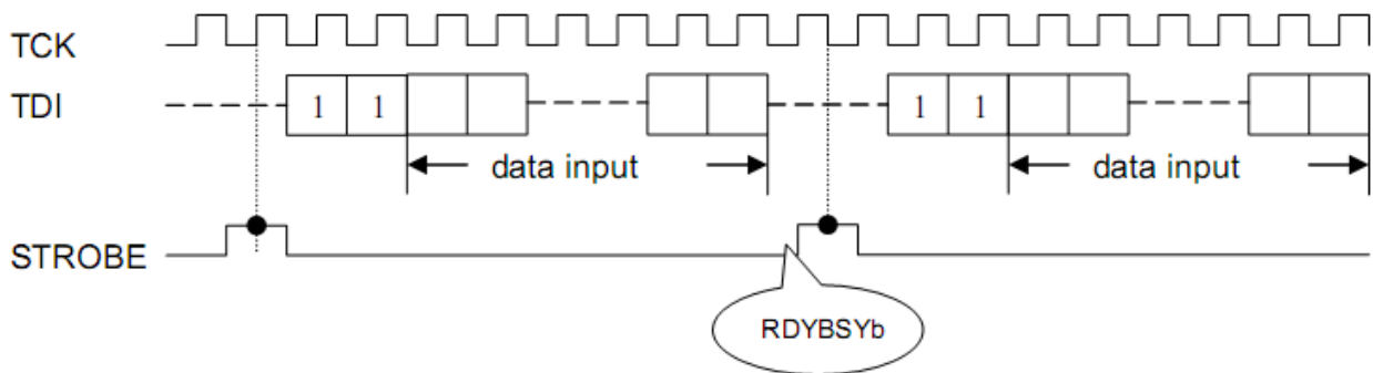
Рисунок 11 – Повтор цикла записи
