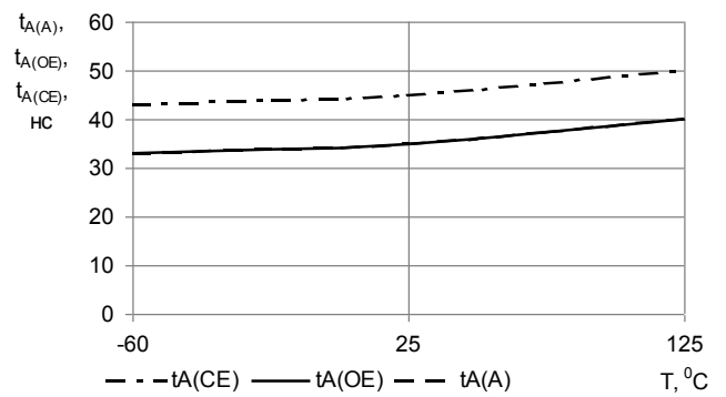
Рисунок 28 – Зависимость времени выборки адреса, t_{A(A)} , времени выборки по сигналу \overline{nCE} , t_{A(nCE)} , времени выборки по сигналу \overline{nOE} , t_{A(nOE)} , от температуры при U_{CC}= 3,0 В
