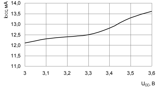
Рисунок 26 – Зависимость динамического тока потребления от напряжения питания при T = - 60 °С
