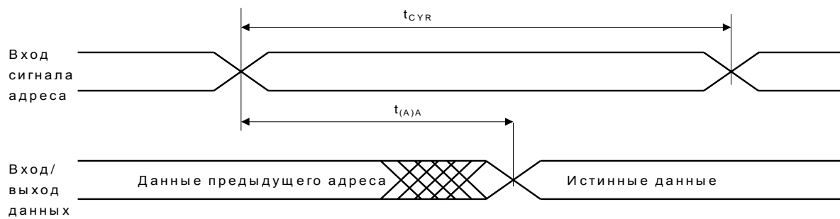
Рисунок 12 – Временная диаграмма цикла чтения 1.
