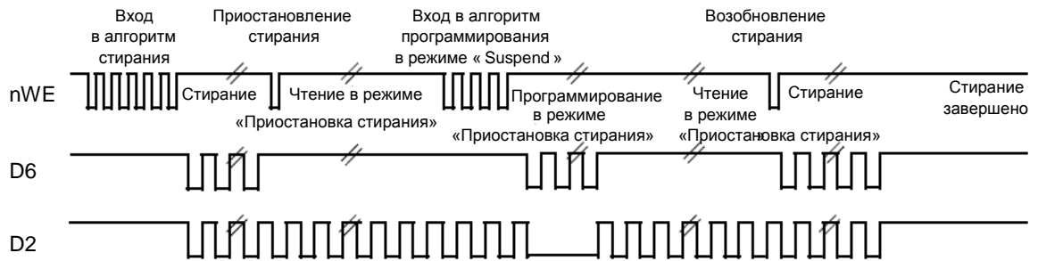
Рисунок 17 – Временная диаграмма переключения статусных бит. Система может использовать nCE или nOE для переключения D2 и D6. D2 переключается только при чтении по адресу внутри стираемого сектора
