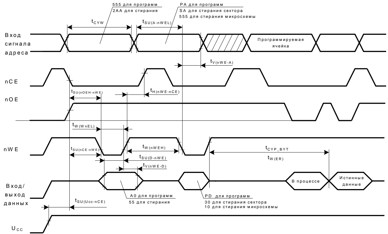
Рисунок 14 – Временная диаграмма цикла записи 1. Управление по nWE. U nOE =U ИН на протяжении цикла записи
