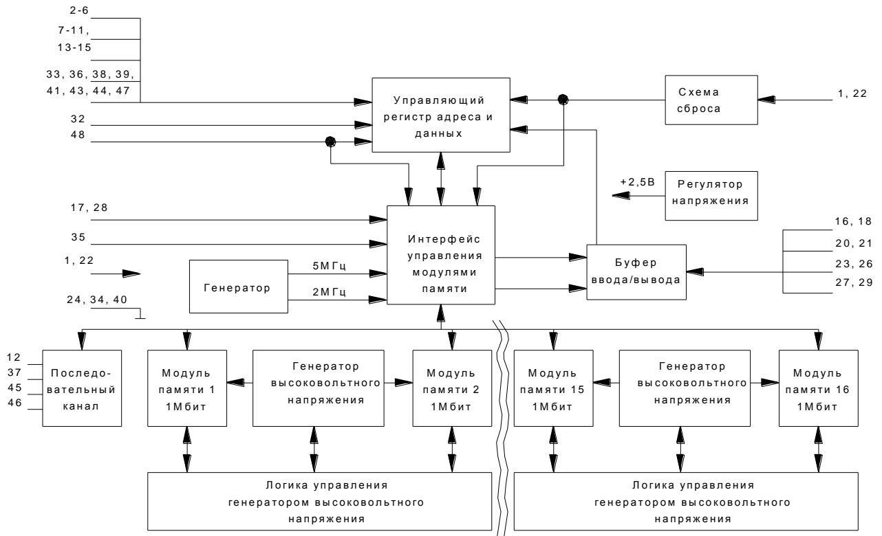
Рисунок 1 – Структурная блок-схема
