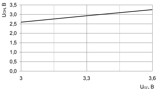
Рисунок 23 – Зависимость выходного напряжения высокого уровня от напряжения питания при I OH = - 4 мА
