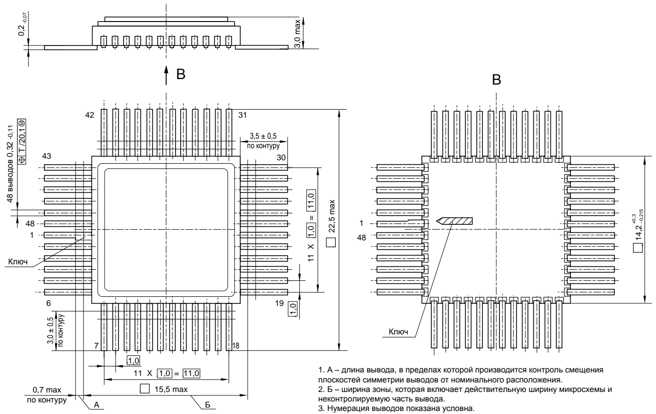
Рисунок 29 – Габаритный чертеж микросхемы в корпусе Н16.48-1В
