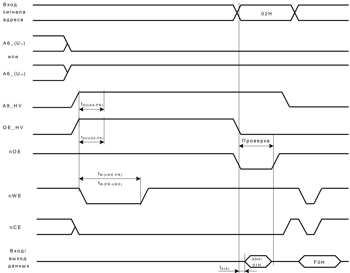
Рисунок 16 – Временная диаграмма цикла защиты/снятия защиты
