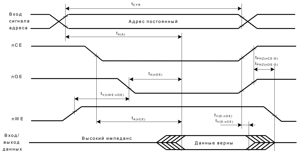
Рисунок 13 – Временная диаграмма цикла чтения 2.
