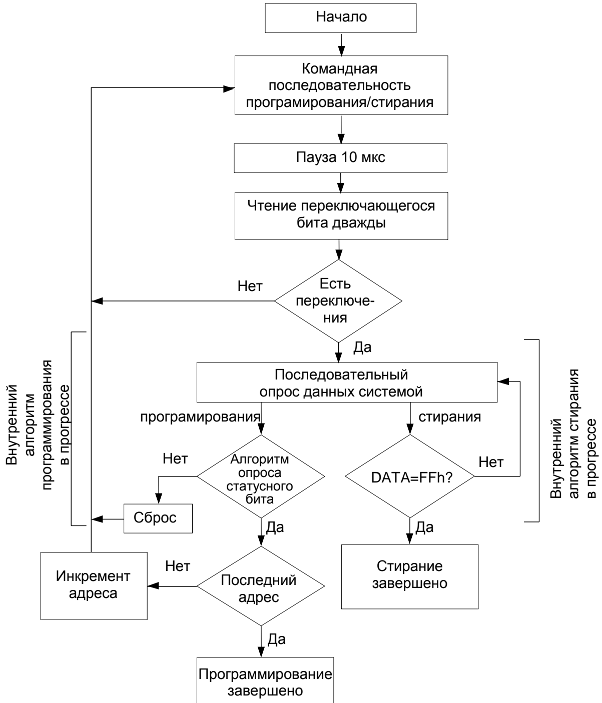
Рисунок 3 – Алгоритм процедуры программирования/стирания
