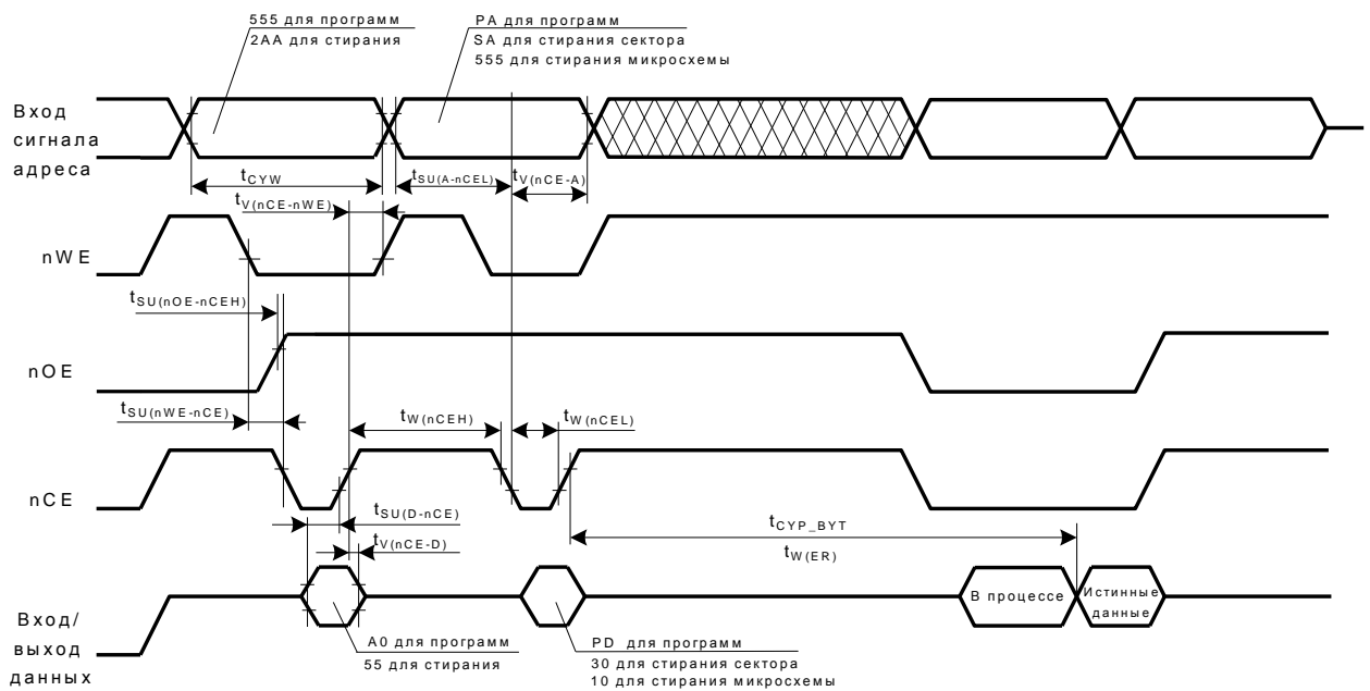
Рисунок 15 – Временная диаграмма цикла записи/стирания 2. Управление по nCE. U nOE =U ИН
