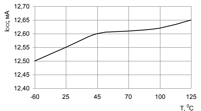
Рисунок 24 – Зависимость динамического тока потребления от температуры при: U CC = 3,3 В, t CYR =120 нс
