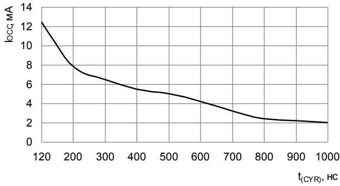
Рисунок 25 – Зависимость динамического тока потребления от времени цикла считывания информации t_{CYR} при: U_{CC}= 3,3 В, T=25 °С
