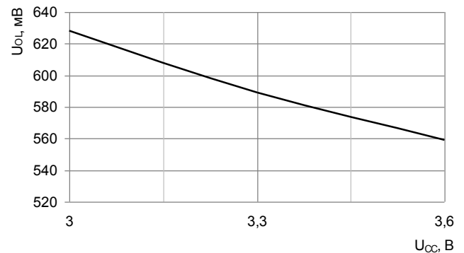
Рисунок 22 – Зависимость выходного напряжения низкого уровня от напряжения питания
