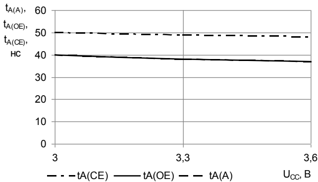
Рисунок 27 – Зависимость времени выборки адреса, t_{A(A)} , времени выборки по сигналу \overline{nCE} , t_{A(nCE)} , времени выборки по сигналу \overline{nOE} , t_{A(nOE)} , от напряжения питания при T= 125 °С
