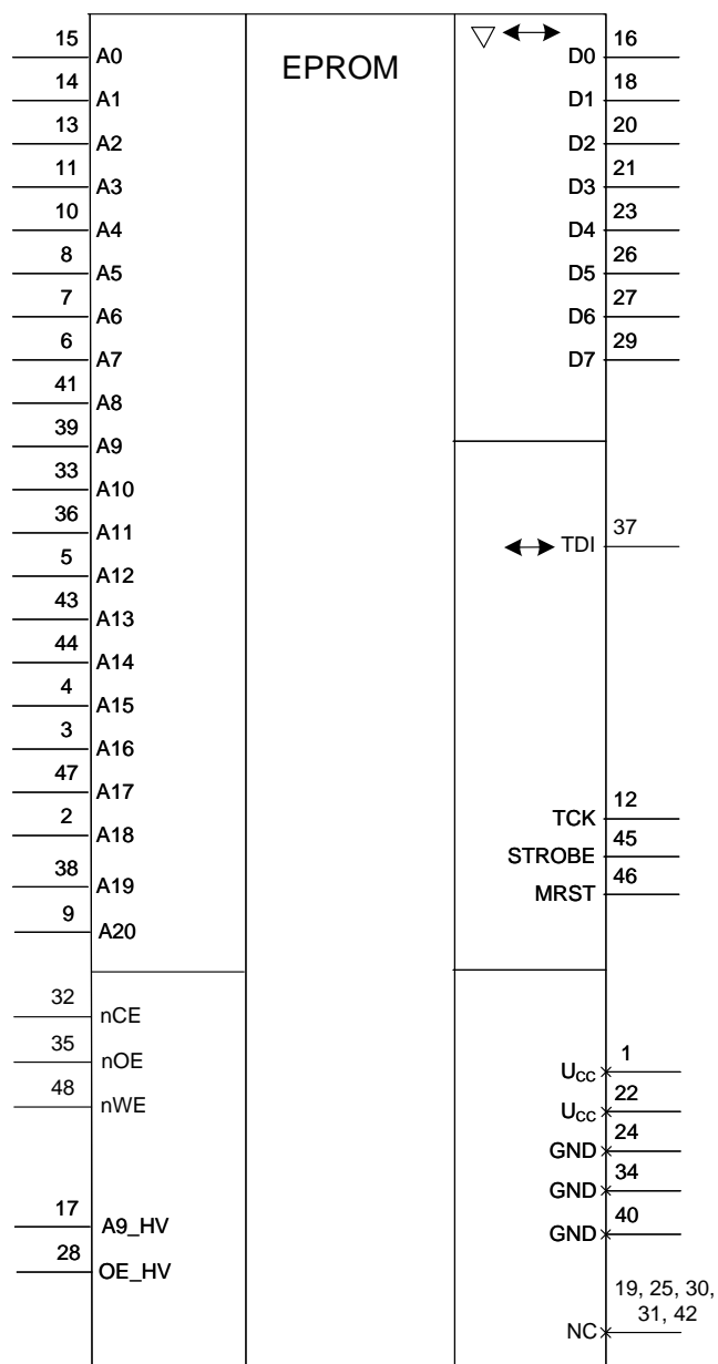
Рисунок 2 – Условное графическое обозначение
