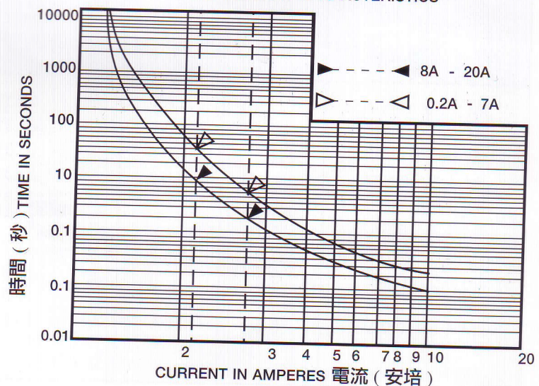
電流時間走勢曲線圖 TIME CURRENT CHARACTERISTICS
