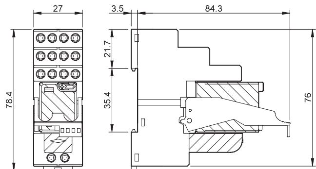
Тип 58.P3 Клеммы Push-in
