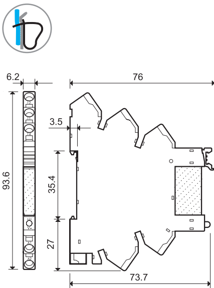
Тип 38.61 / 38.61.3 38.91 / 38.91.3 Пружинный клеммы
