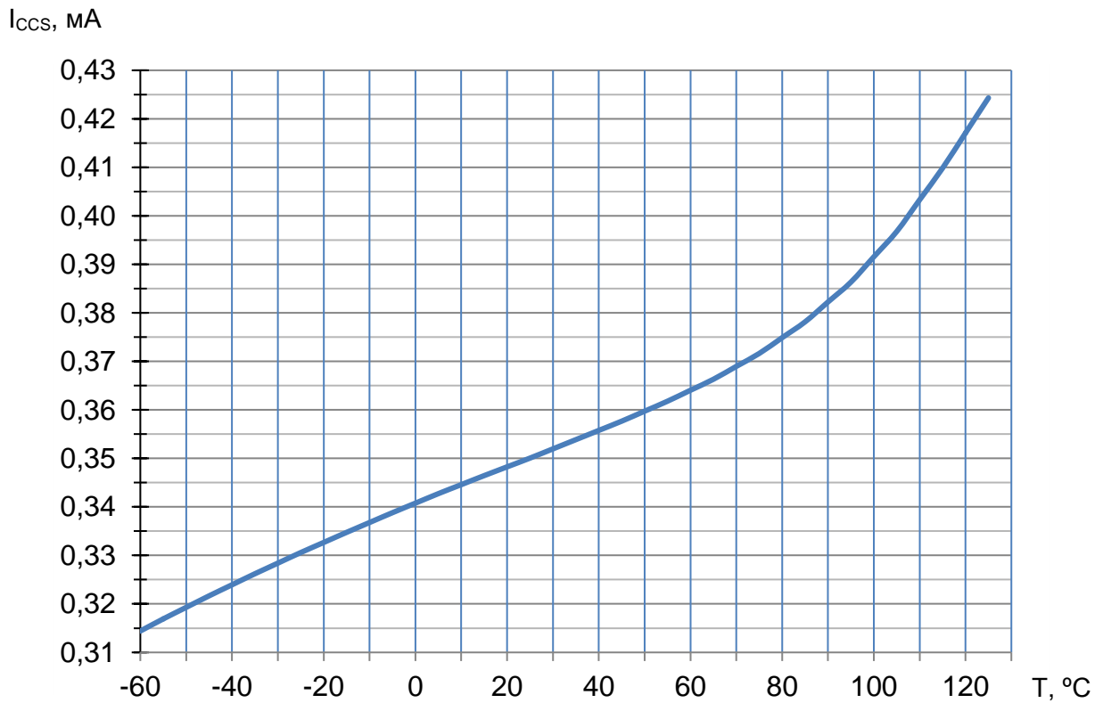
Рисунок 38 – Зависимость тока потребления в режиме хранения от температуры при U in = 3,6 В
