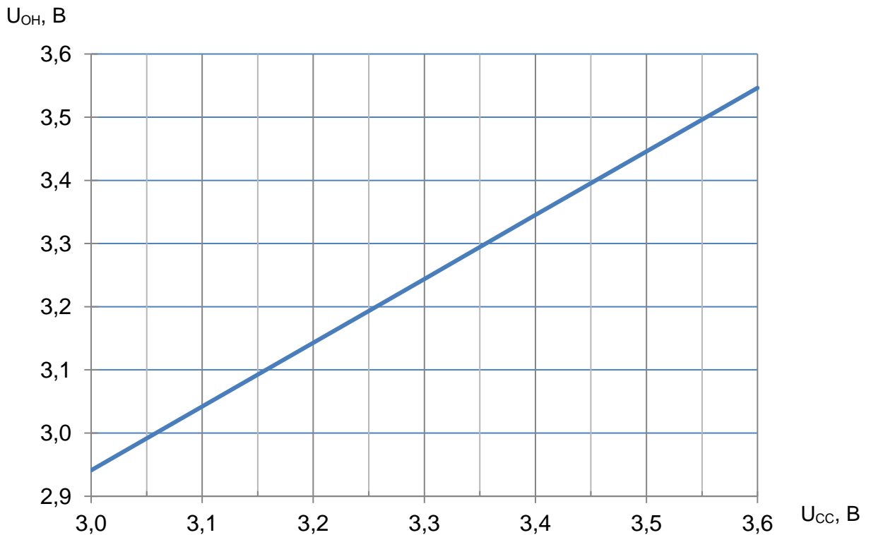
Рисунок 42 – Зависимость выходного напряжения высокого уровня от напряжения питания при I_{OH} = минус 2 мА, T = 25 °С
