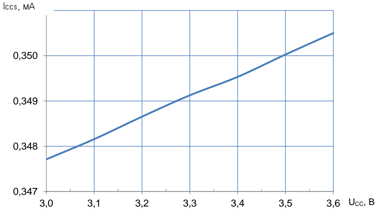
Рисунок 37 – Зависимость тока потребления в режиме хранения от напряжения питания при T = 25 °C
