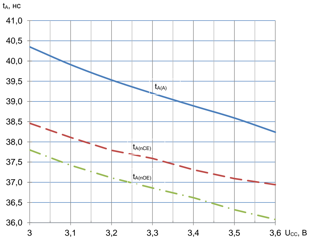
Рисунок 46 – Зависимость времени выборки адреса, t_{A(A)} , времени выборки по сигналу nCE, t_{A(CE)} , времени выборки по сигналу nOE, t_{A(OE)} от напряжения питания при T = 125 °C
