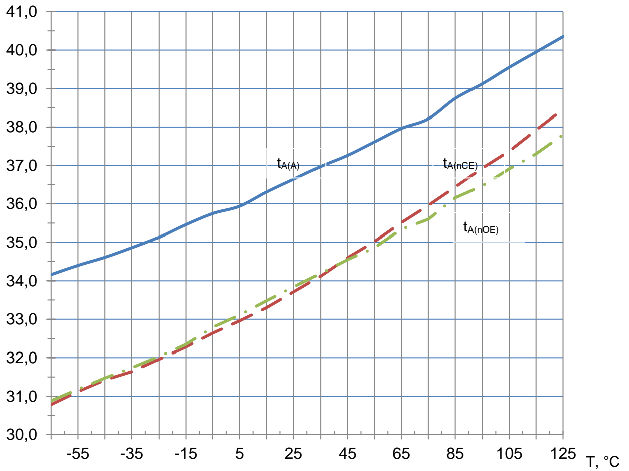
Рисунок 47 – Зависимость времени выборки адреса, t_{A(A)} , времени выборки по сигналу nCE, t_{A(nCE)} , времени выборки по сигналу nOE, t_{A(nOE)} от температуры при U_{CC} = 3,0 В
