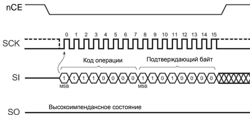
Рисунок 26 – Операция сброса
