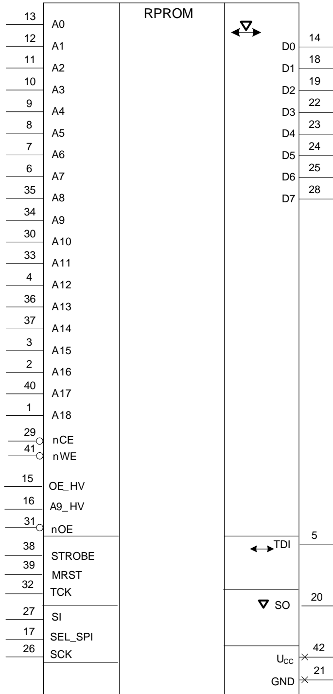
Рисунок 2 – Условно-графическое обозначение
