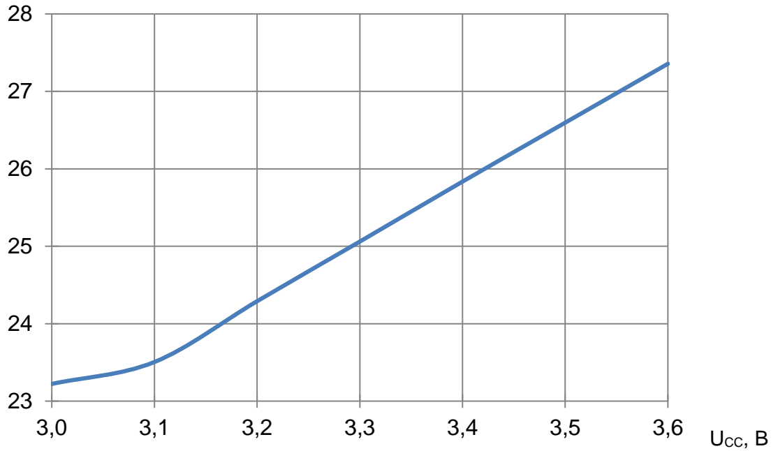
Рисунок 45 – Зависимость динамического тока потребления от напряжения питания при t_{CYR} = 65 нс, T = -60 °C
