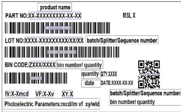
Fig. 2-3 Label 标签
