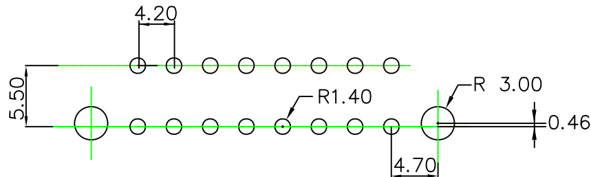
P.C.Board layout
