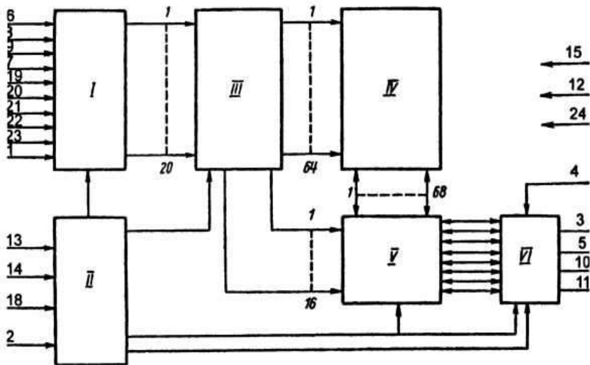
Структурная схема КР1601РР1:
