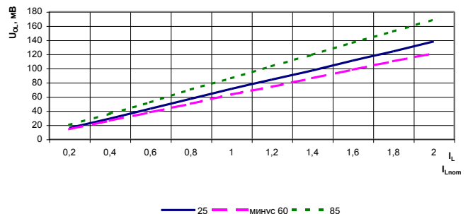
Рисунок 17 – Зависимость выходного напряжения низкого уровня цифровых выходов link_rec[3:0], partition[3:0], collision, chain_o, request_n, data_bus, U_{OL} , от тока нагрузки, при T = 25^\circ \text{С} , T = 125^\circ \text{С} , T = \text{минус } 60^\circ \text{С} , |I_{Lnom}| = 6 \text{ мА}
