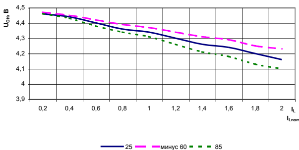
Рисунок 16 – Зависимость выходного напряжения высокого уровня цифровых выходов link_rec[3:0], partition[3:0], collision, chain_o, request_n, data_bus, U_{OH} , от изменения тока нагрузки, при T = 25^\circ \text{С} , T = 125^\circ \text{С} , T = \text{минус } 60^\circ \text{С} , |I_{Lnom}| = 6 \text{ мА}
