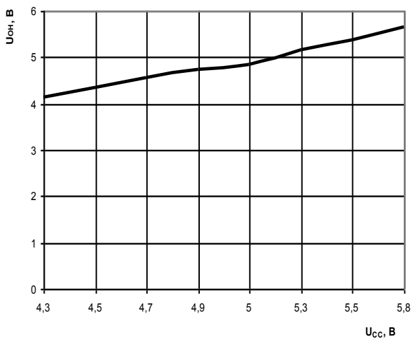
Рисунок 10 – Зависимость выходного напряжения высокого уровня цифровых выходов link_rec[3:0], partition[3:0], collision, chain_o, request_n, data_bus, U он , от напряжения питания U cc , при I OL =минус 6 мА, T=25°С
