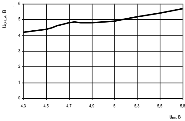
Рисунок 12 – Зависимость выходного напряжения высокого уровня аналоговых выходов txdp[3:0], txdm[3:0], dtrop[3:0], dtrom[3:0], xt2, U_{OH\_A} , от напряжения питания U_{CC} , при I_{OL} = \text{минус } 6 \text{ мА} , T = 25^\circ \text{С} питания, при I_L = 6 \text{ мА}
