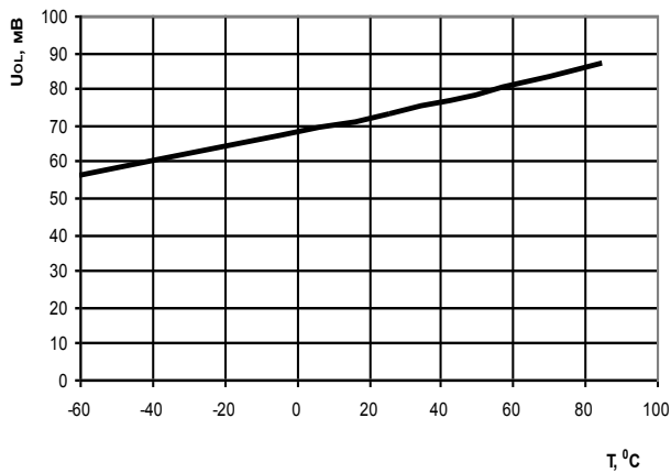
Рисунок 6 – Зависимость выходного напряжения низкого уровня аналоговых выходов txdp[3:0], txdm[3:0], dtpop[3:0], dtprom[3:0], xt2, U OL_A , от температуры T°, при I OL =6 мА
