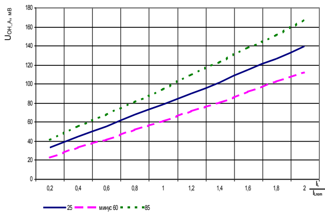
Рисунок 18 – Зависимость выходного напряжения высокого уровня аналоговых выходов txdp[3:0] , txdm[3:0] , dtrp[3:0] , dtrpm[3:0] , xt2 , U_{OL\_A} , от тока нагрузки, при T=25\text{ }^{\circ}\text{C} , T=125\text{ }^{\circ}\text{C} , T=\text{минус } 60\text{ }^{\circ}\text{C} , |I_{Lnom}|=6\text{ mA}
