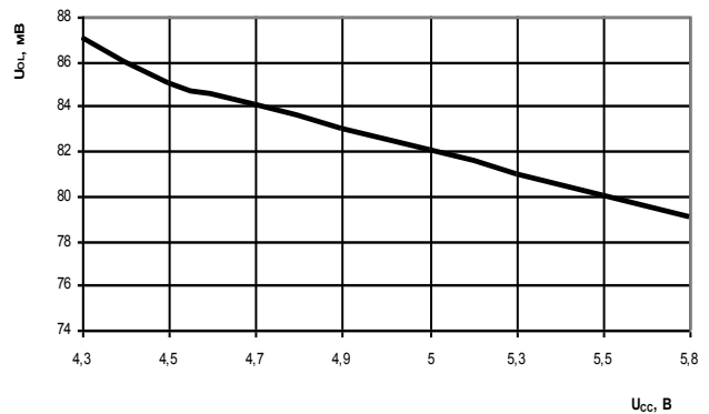
Рисунок 11 – Зависимость выходного напряжения низкого уровня цифровых выходов link_rec[3:0], partition[3:0], collision, chain_o, request_n, data_bus, U ол , от напряжения питания U cc , при I OL =6 мА, T=25°С
