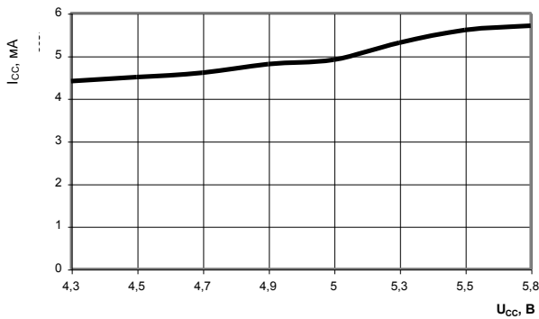
Рисунок 14 – Зависимость статического тока потребления I_{CC} от напряжения питания U_{CC} при T = 25^\circ \text{С}
