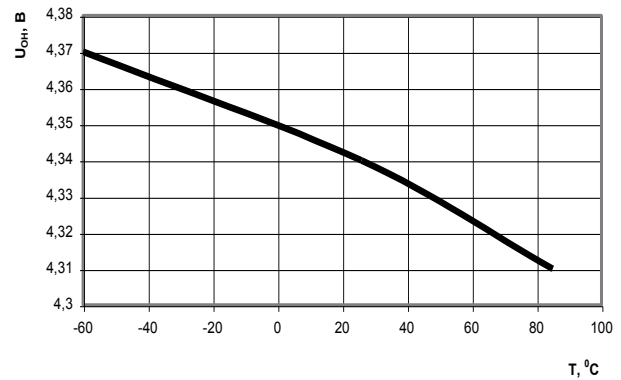
Рисунок 5 – Зависимость выходного напряжения высокого уровня цифровых выходов link_rec[3:0], partition[3:0], collision, chain_o, request_n, data_bus, U OH , от температуры T°, при I OL =минус 6 мА
