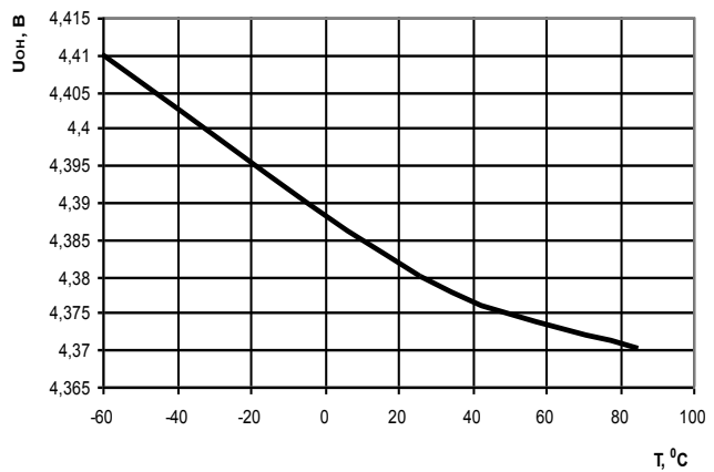
Рисунок 7 – Зависимость выходного напряжения высокого уровня аналоговых выходов txdp[3:0], txdm[3:0], dtpop[3:0], dtprom[3:0], xt2, U OH_A , от температуры T°, при I OL =минус 6 мА
