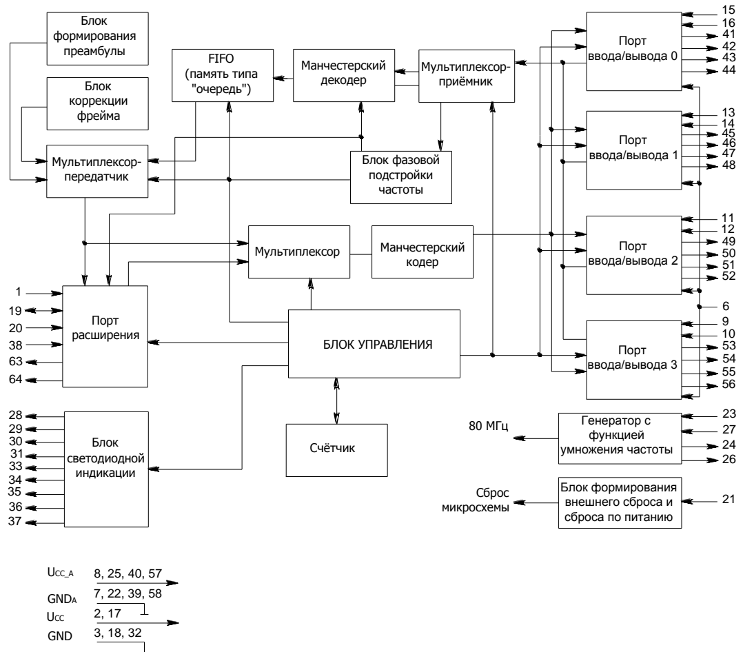
Рисунок 1 – Структурная блок-схема
