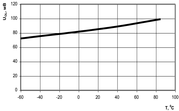
Рисунок 4 – Зависимость выходного напряжения низкого уровня цифровых выходов link_rec[3:0], partition[3:0], collision, chain_o, request_n, data_bus, U OL , от температуры T°, при I OL =6 мА
